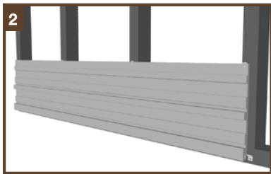
การเกี่ยวคิลิปล็อกกับ ร่องด้านล่างแผ่น
