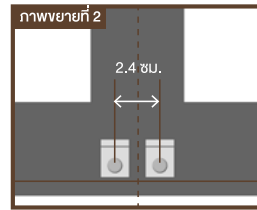
แสดงลักษณะการติดคิลิปล็อกบริเวณรอยต่อแผ่นไม้
